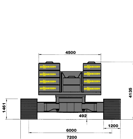
mit Laufwerk B9HD 8800 mm Länge - with crawler B9HD 8800 mm length
